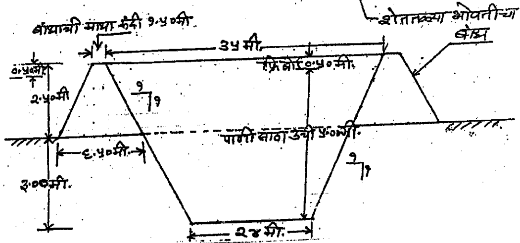
शेततळ्याचा काटछेद
