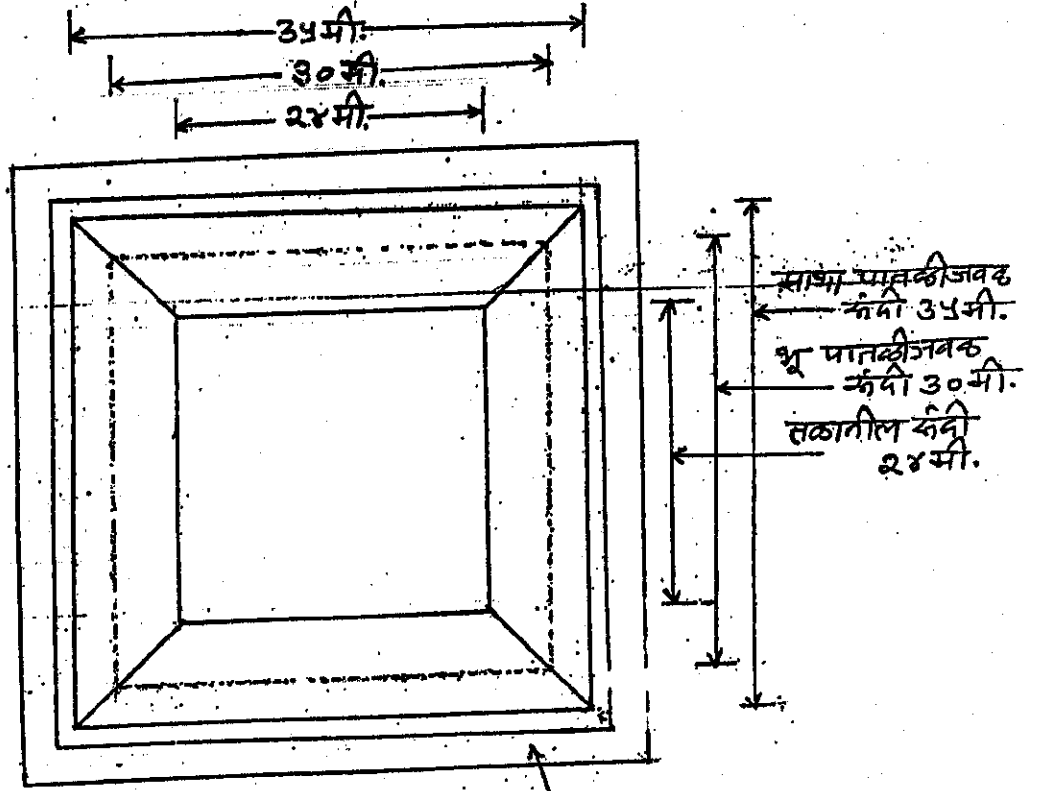
शेततळ्याचा प्लॅन
